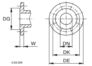
Фланцы PN 10, EN 1092-2
